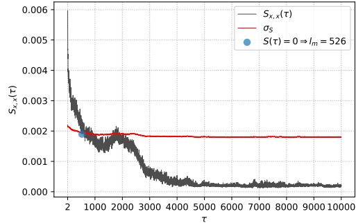
(آ) در این شکل S_1 نشان دهنده طول مارکوف بیتکوین به خودش است، l_1 = 526 .
