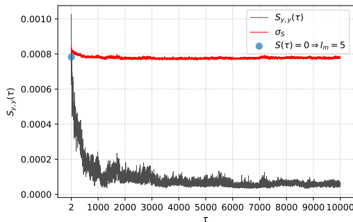
(د) در این شکل S_4 نشان دهنده طول مارکوف اتریوم به خودش است، l_4 = 5 .
