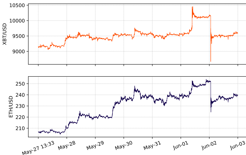
شکل ۳.۴: قیمت قراردادهای دائمی بیتکوین و اتریوم بر حسب دلار آمریکا در بازه شماره ۱.
