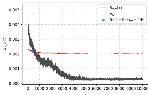
(د) در این شکل S_4 نشان دهنده طول مارکوف اتریوم به خودش است، l_4 = 436 .
