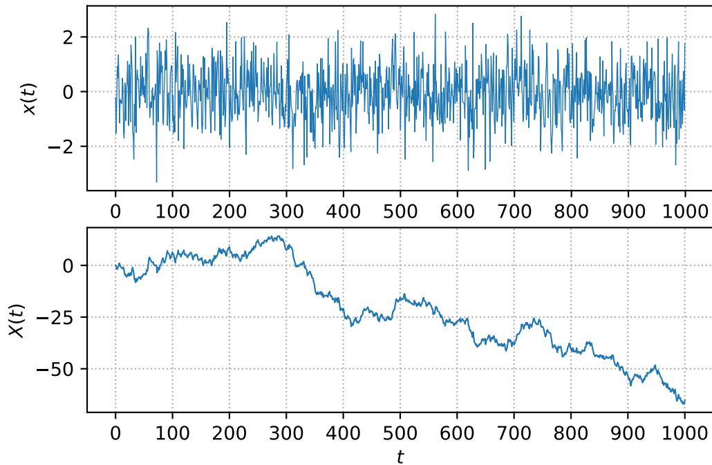
شکل ۸.۲: یک نمونه از فرایند تصادفی که با استفاده از رابطه ۵۹.۲ با p = 18 تولید شده است. در این شکل X_{t+1} = X_t + x_t است.
