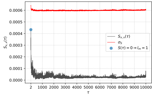
(آ) در این شکل S_1 نشان دهنده طول مارکوف بیتکوین به خودش است، l_1 \leq 1 .
