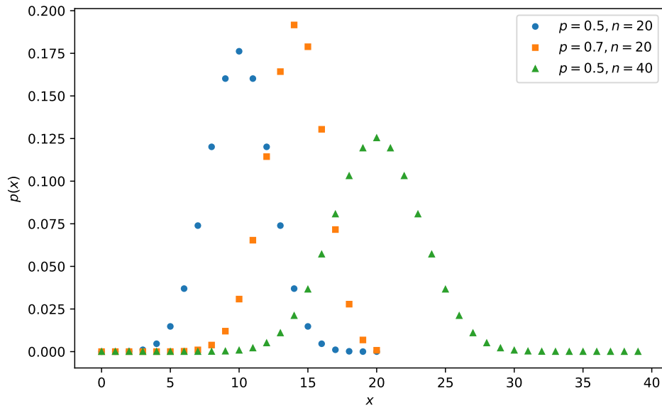
شکل ۳.۱: چند نمونه از توزیع دو جمله‌ای
