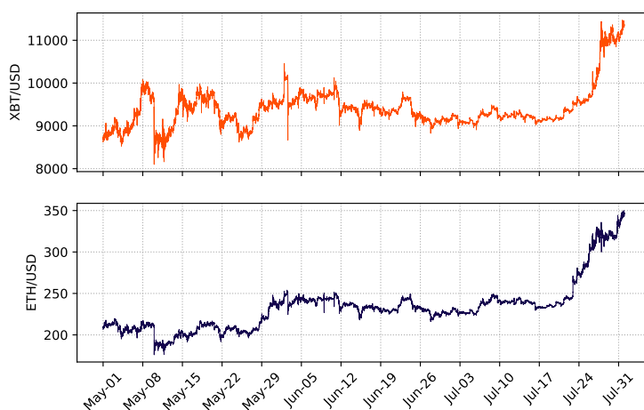
شکل ۱.۴: قیمت قراردادهای دائمی بیتکوین و اترיום بر حسب دلار آمریکا در صرافی بیتمکس در بازه سه ماهه می تا جولای ۲۰۲۰.
