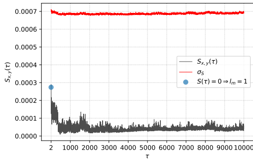
(ب) در این شکل S_2 نشان دهنده طول مارکوف بیتکوین به اتریوم است، l_2 \leq 1 .
