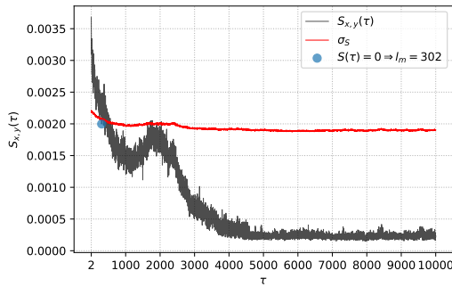
(ب) در این شکل S_2 نشان دهنده طول مارکوف بیتکوین به اتریوم است، l_2 = 302 .
