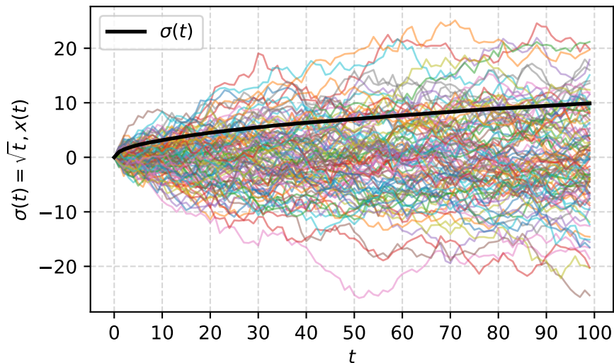
شکل ۲.۲: چند نمونه مستقل از فرایند ولگشت تصادفی که قدمهایی با توزیع گاوسی برمی دارد.
