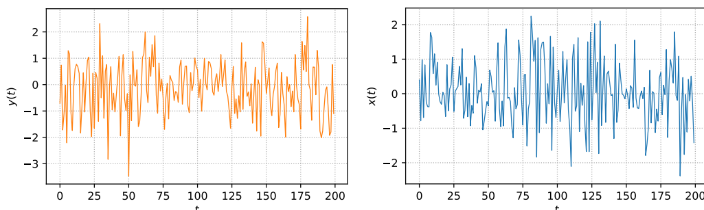
(ب) فرایند y با l_3 = 15 , l_4 = 25 .
