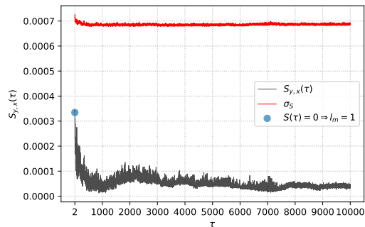
(ج) در این شکل S_3 نشان دهنده طول مارکوف اتریوم به بیتکوین است، l_3 \leq 1 .
