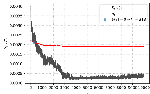
(ج) در این شکل S_3 نشان دهنده طول مارکوف اتریوم به بیتکوین است، l_3 = 313 .
