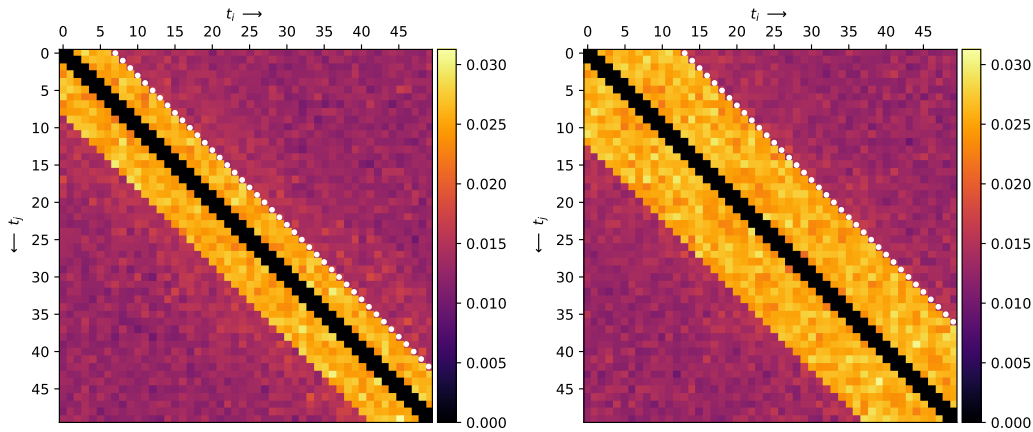
شکل ۵.۳: نمودار S_1(t_i, t_j) و S_2(t_i, t_j) که نشان دهنده وابستگی فرایند x به خودش و به فرایند y هستند.
